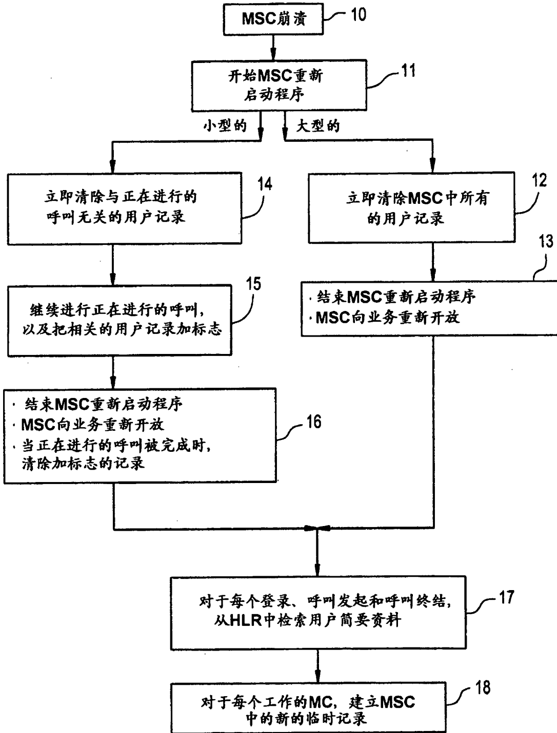
图 1 现有技术
